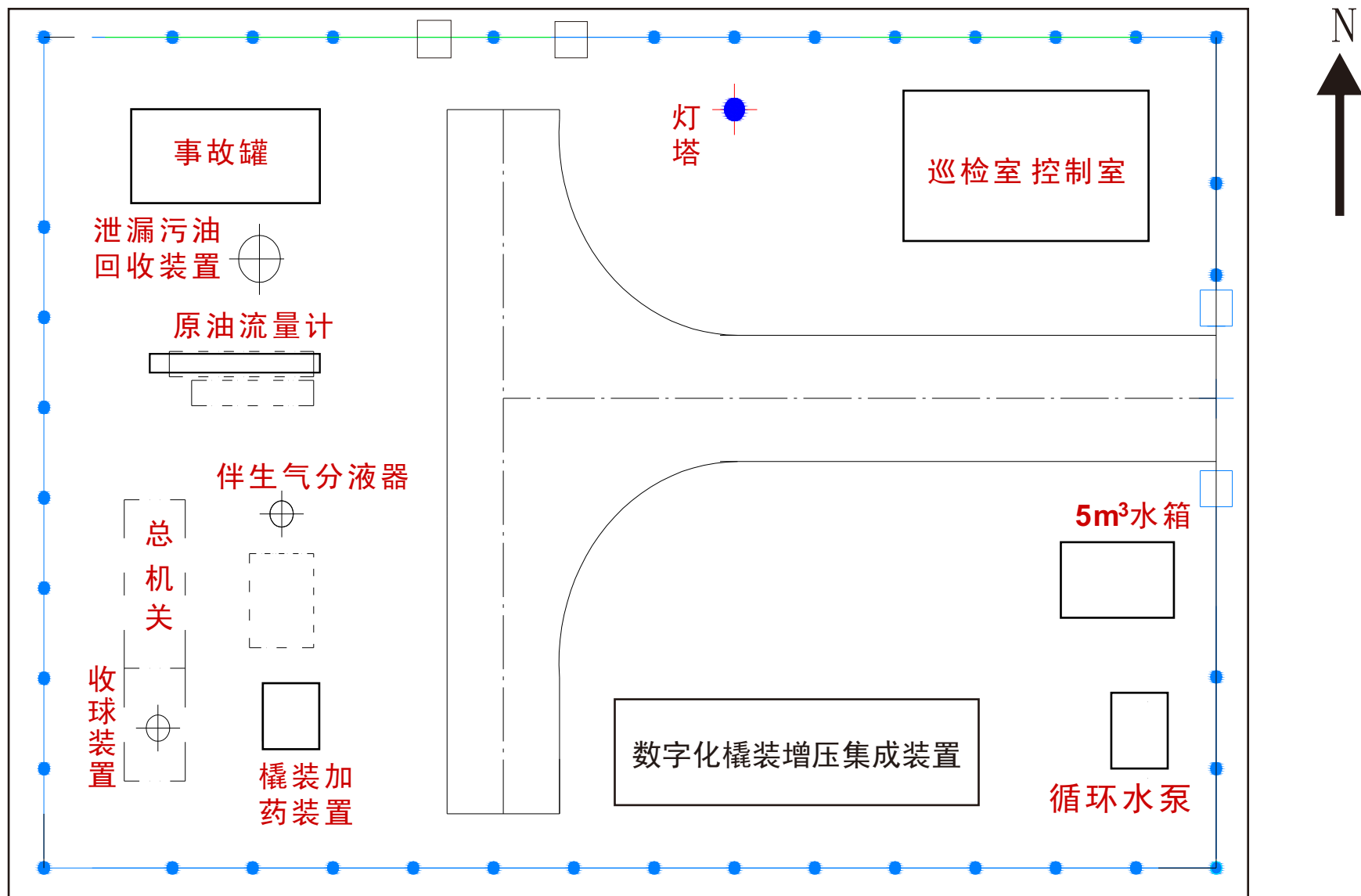
薛9增平面布置示意图
